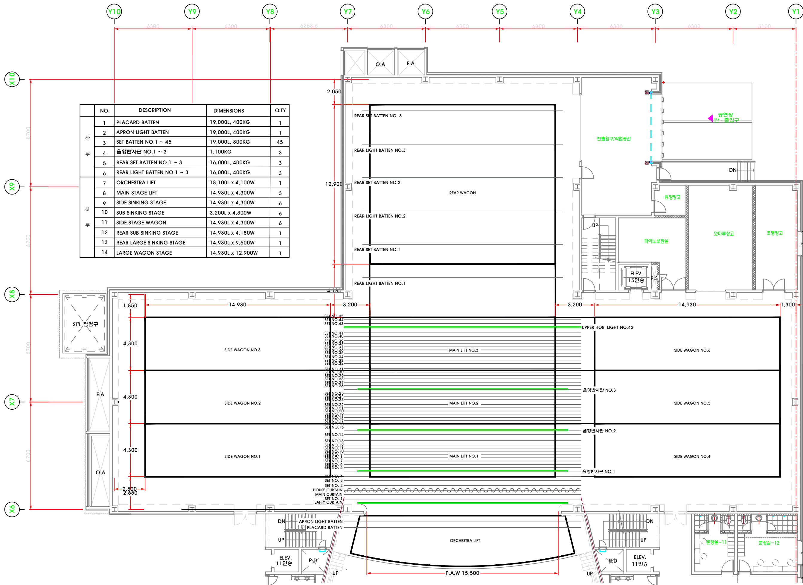
무대기계 평면도
